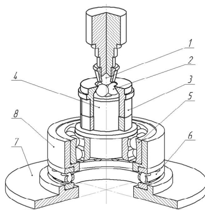
Рис. 1 – Робочий вузол установки для чотирикулькової схеми
